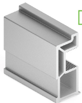
AV0793.VP540.SLMAN.CJ Профиль верт. SLIM MAX, L=5400, Серебро матовое
