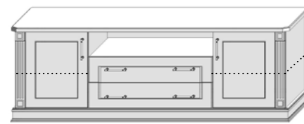
Yv.TTV.O-1 □ 1684 □ 575 □ 490
