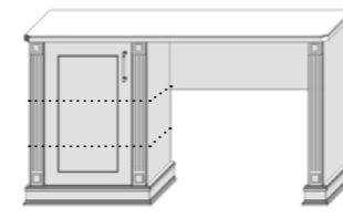
Yv.TS.O-1 □ 1310 □ 731 □ 430
