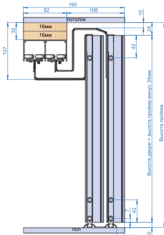
Скрытая установка направляющей верхней в проём
